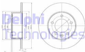
TARCZA HAM RENAULT MASTER 10> TYŁ L/P 2.3 DCI
